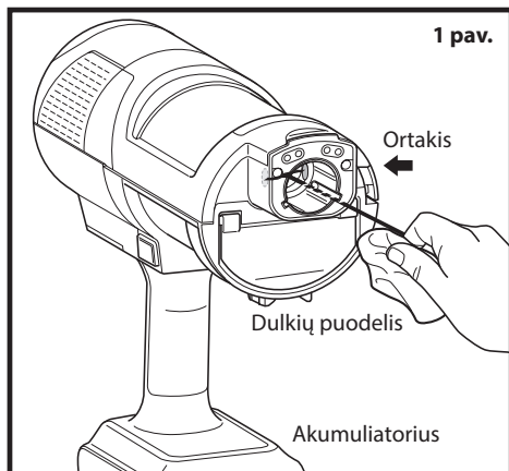
NEŠVARUMŲ APTIKIMO JUTIKLIAI
